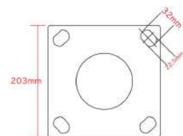
設置プレートサイズ(全種共通)
